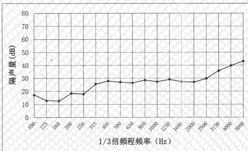
试件的隔声特性曲线图
